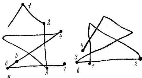
Рис. 1. Графический рисунок «конверта», выполненный испытуемым не глядя на руку a — первая проба; б — четвертая проба; точками и цифрами обозначены последовательные моменты появления быстрых фаз ФОКН
